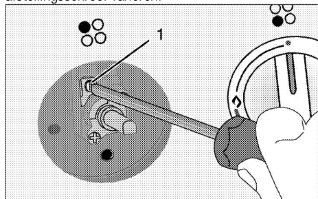
1 Stelschroef gasdebiet
