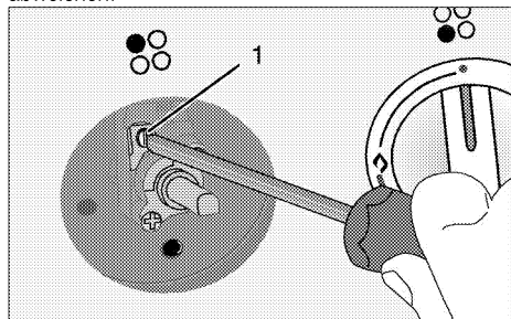
1 Gasdurchfluss-Einstellschraube
