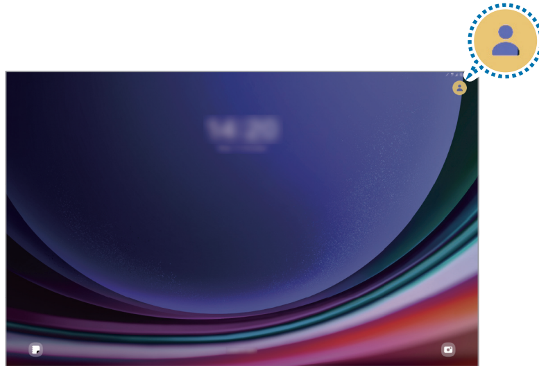
Vergrendelscherm
